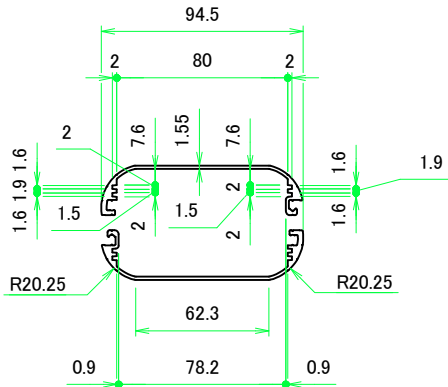
本体フレーム1 Frame 1
