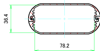
A-A (1:2)
